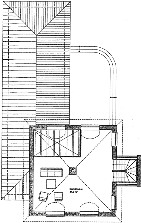
Tagetage 1:100
